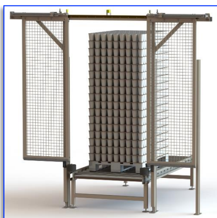
Abbildung 1: Maschinenschutzschiebetür offen
